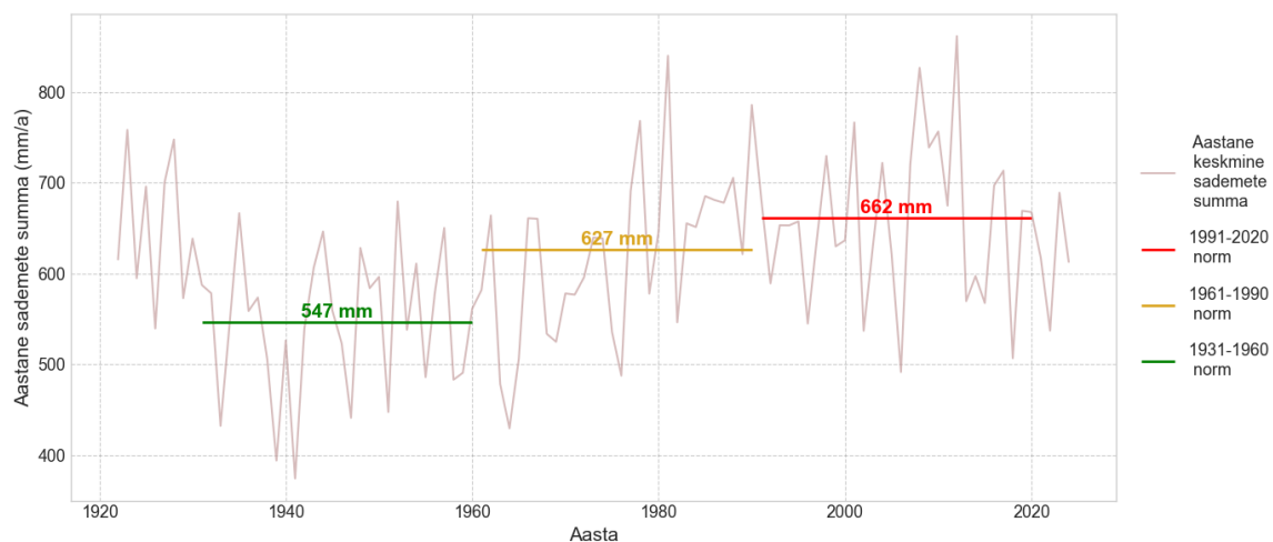
Joonis 3: Eesti aastaste keskmiste sademete summa aegrida. Adapteeritud Keskkonnaportaalist. Andmed Keskkonnaagentuurist.
