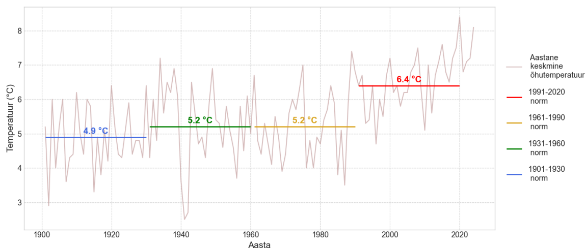
Joonis 2: Eesti aastaste keskmiste temperatuuride aegrida. Adapteeritud Keskkonnaportaalist. Andmed Keskkonnaagentuurist.
