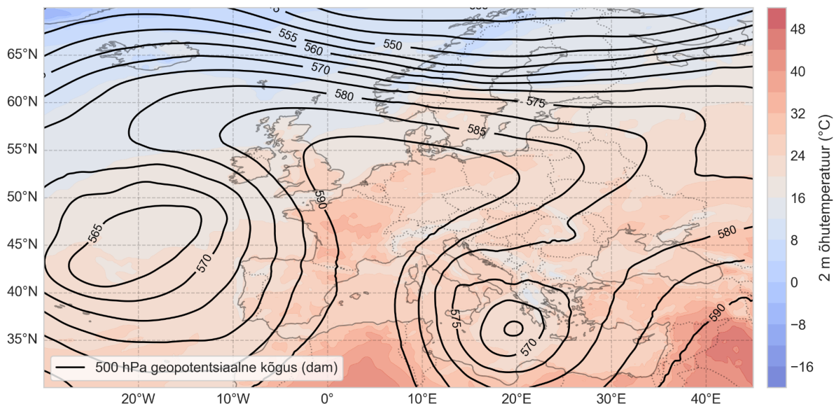
Joonis 6: Euroopa 500 hPa geopotentsiaalse kõrguse ja 2 m õhutemperatuuri kaart (19.06.2025 12:00). Andmed: ERA5
